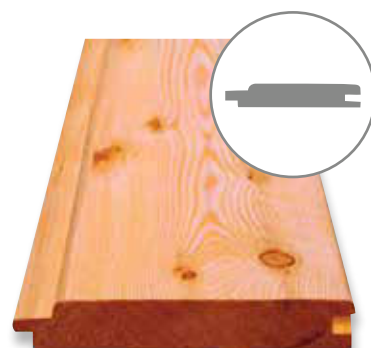
Rundkantenprofil im Schnitt: 19,5 x 96 mm mit Nut und Feder. Bsp. zeigt „Natur“ (Lärche).
