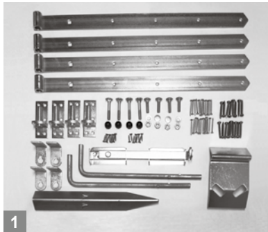
1 Für: Doppeltore mit geradem Riegel Inhalt: 4 gerade Ladenbänder 16 x 700 mm, 4 Kloben, 1 Do.-Überwurf, 2 Bodenschieber, 1 Auflaufstütze mit abschraubbarem Erddorn, 1 Schraubensortiment. Passend z. B. für Doppeltor Usedom, Holsteinzaun etc.
