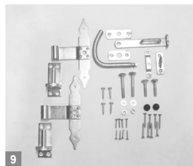
9 Für: Bogen-Dichtzauntüren (auch für gerade Türen verwendbar) Inhalt: 2 Kreuzbänder/Mittelbänder mit Zierspitze, 2 Kloben, 1 „dänischer“ Türverschluss, 1 Schraubensortiment. Passend z. B. für Monegro, Sontegro.
