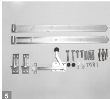
5 Für: schwere Einzeltore und Pforten mit geradem Riegel Inhalt: 2 gerade Ladenbänder 16 x 600 mm, 2 Kloben, 1 Gartentorfaller, 1 Schraubensortiment. Passend z. B. für Pforten Usedom, Holsteinzaun, Staketenzaun etc.
