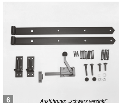
6 Ausführung: „schwarz verzinkt“ Für: schwere Einzeltore und Pforten mit geradem Riegel Inhalt: 2 gerade Ladenbänder 16 x 600 mm, 2 Kloben, 1 Gartentorfaller, 1 Schraubensortiment. Passend z. B. für Pforten Usedom, Holsteinzaun, Staketenzaun etc.
