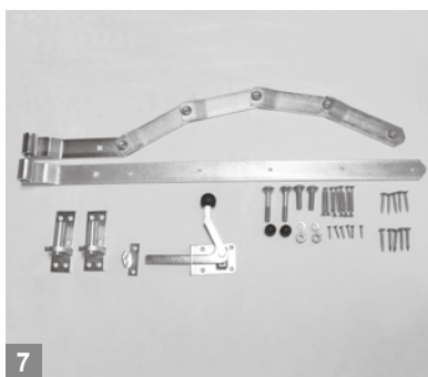
7 Für: Pforten mit gebogenem Riegel Inhalt: 1 gerades Ladenband gekröpft u. 1 verstellb. Bogenladenband 16 x 800 mm inkl. 2 Kloben, 1 Gartentorfaller, 1 Schraubensortiment.
