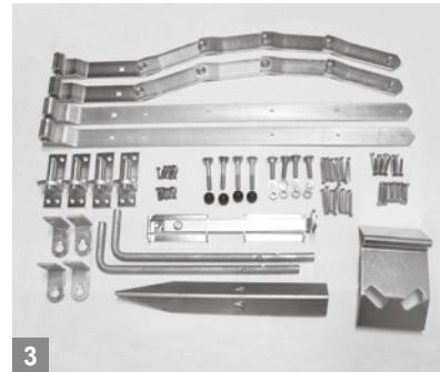
3 Für: Doppeltore mit gebogenem Riegel Inhalt: 2 gerade u. 2 verstellb. Bogenladenbänder 16 x 800 mm, 4 Kloben – verstellbar von 5-23 mm, 1 Do.-Überwurf, 2 Bodenschieber, 1 Auflaufstütze mit abschraubbarem Erddorn, 1 Schraubensortiment. Passend z. B. für Doppeltor Norderney etc.
